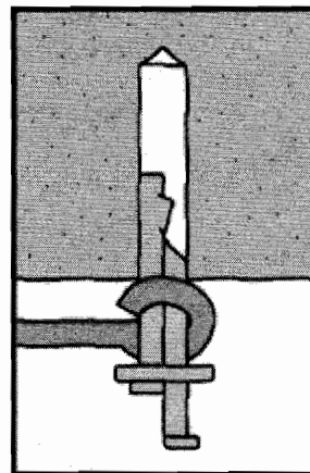
Dübel durch das Anbauteil in das Bohrloch stecken
