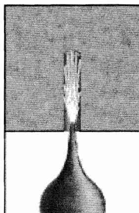
Bohrlochreinigung durch Ausblasen
