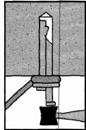
Spreizteil bündig durch Hammerschläge eintreiben
